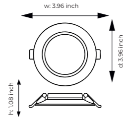
D: 100.5 mm H: 27.5 mm W: 100.5 mm w: 3.96 inch d: 3.96 inch h: 1.08 inch
