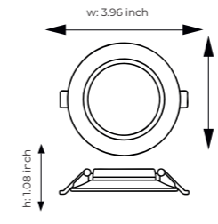
D: 100.5 mm H: 27.5 mm W: 100.5 mm
