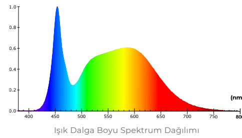
Işık Dalga Boyu Spektrum Dağılımı
