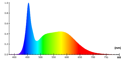
ışık Dalga Boyu Spektrum Dağılımı
