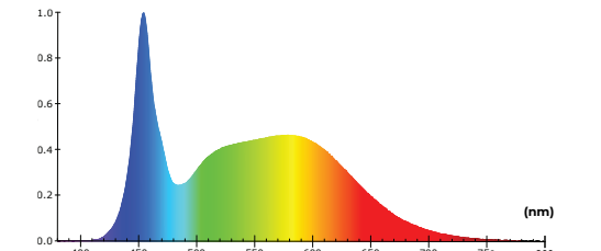
Işık Dalga Boyu Spektrum Dağılımı
