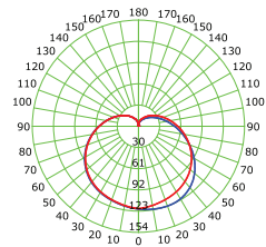
Işık Dağılım Diyagramı
