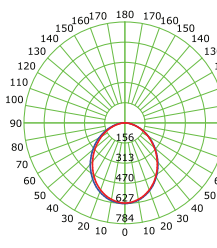
Işık Dağılım Diyagramı
