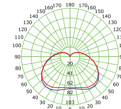
Işık Dağılım Diyagramı
