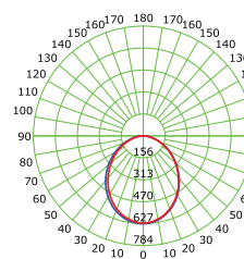
Işık Dağılım Diyagramı
