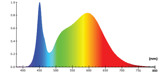
Işık Dalga Boyu Spektrum Dağılımı
