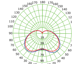
Işık Dağılım Diyagramı
